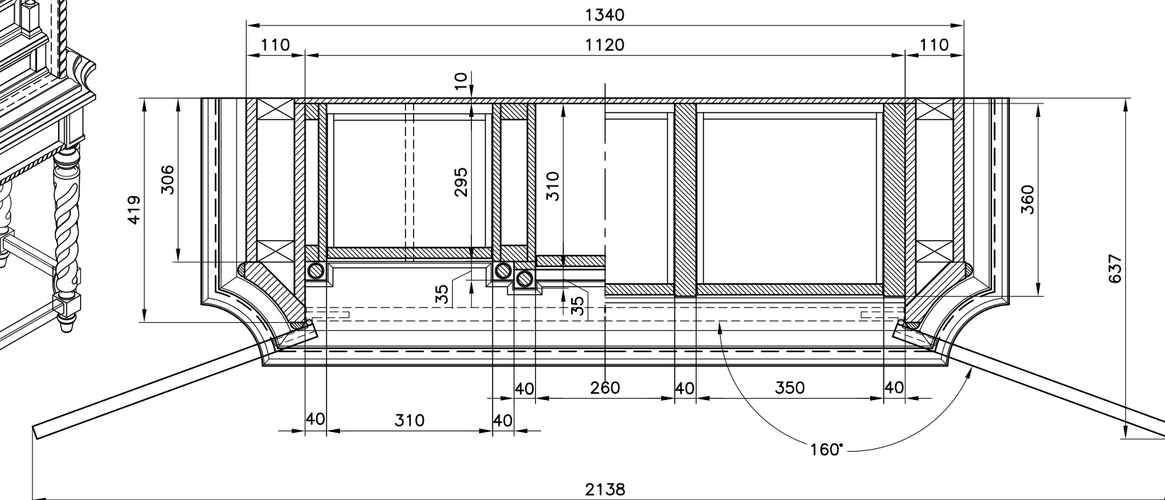
SEZIONE E-E
