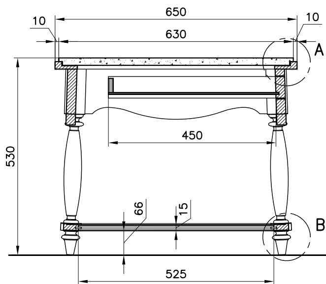
SEZIONE VERTICALE
