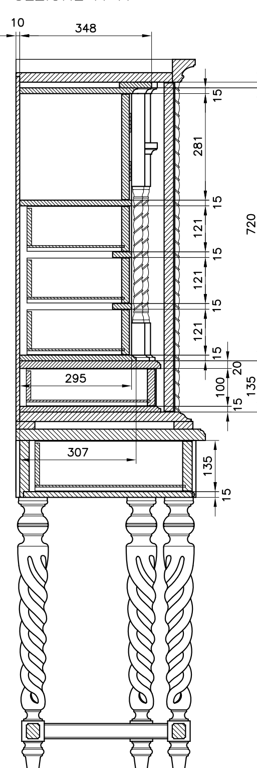
SEZIONE A-A
