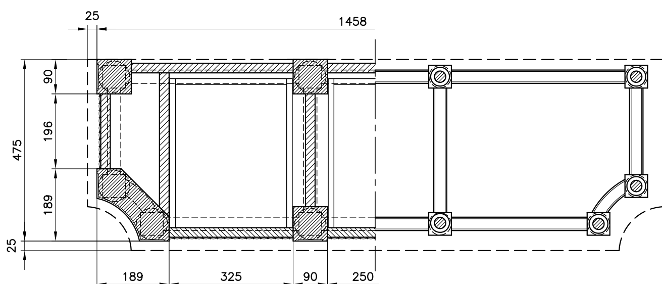
SEZIONE C-C
