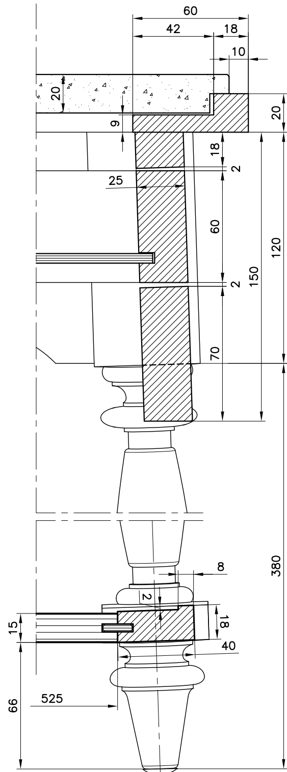
PARTICOLARE A-B scala 1:2
