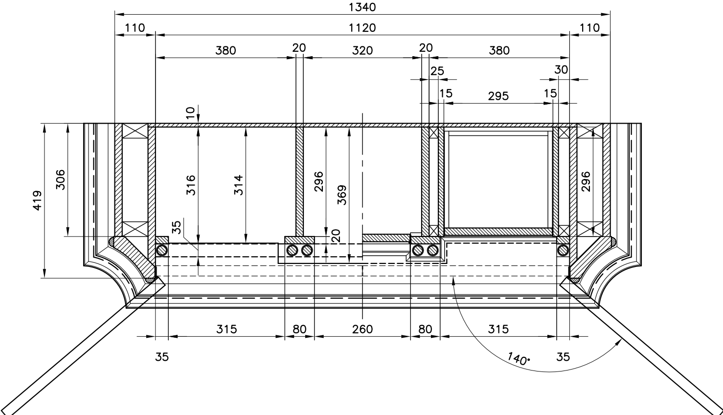
SEZIONE E-E
