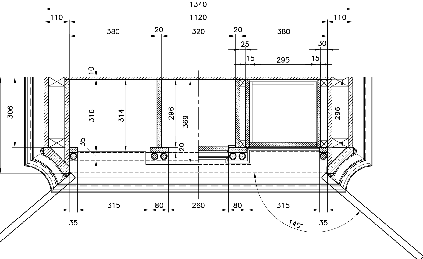
SEZIONE E-E
