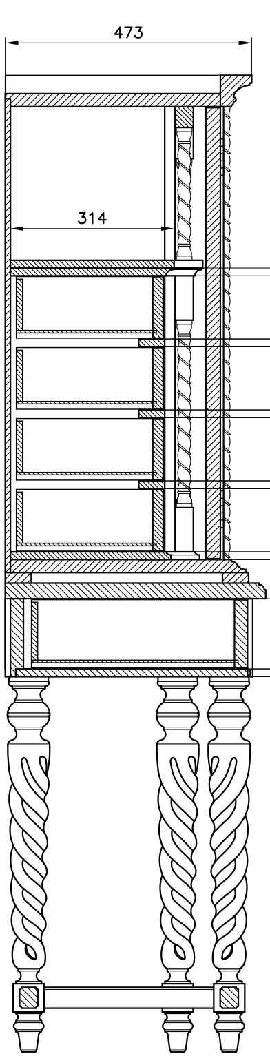
SEZIONE A-A
