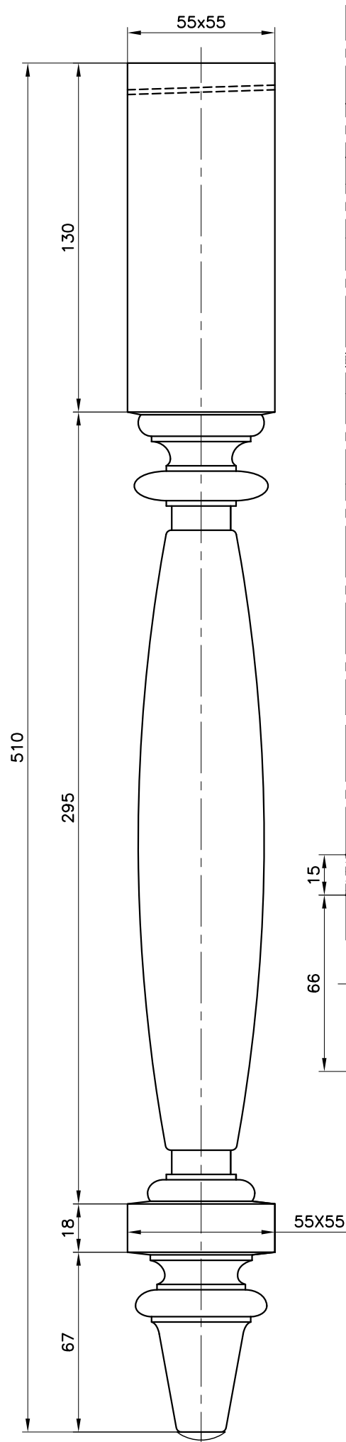
VISTA GAMBA scala 1:2
