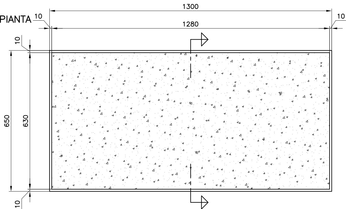
SEZIONE ORIZZ.
