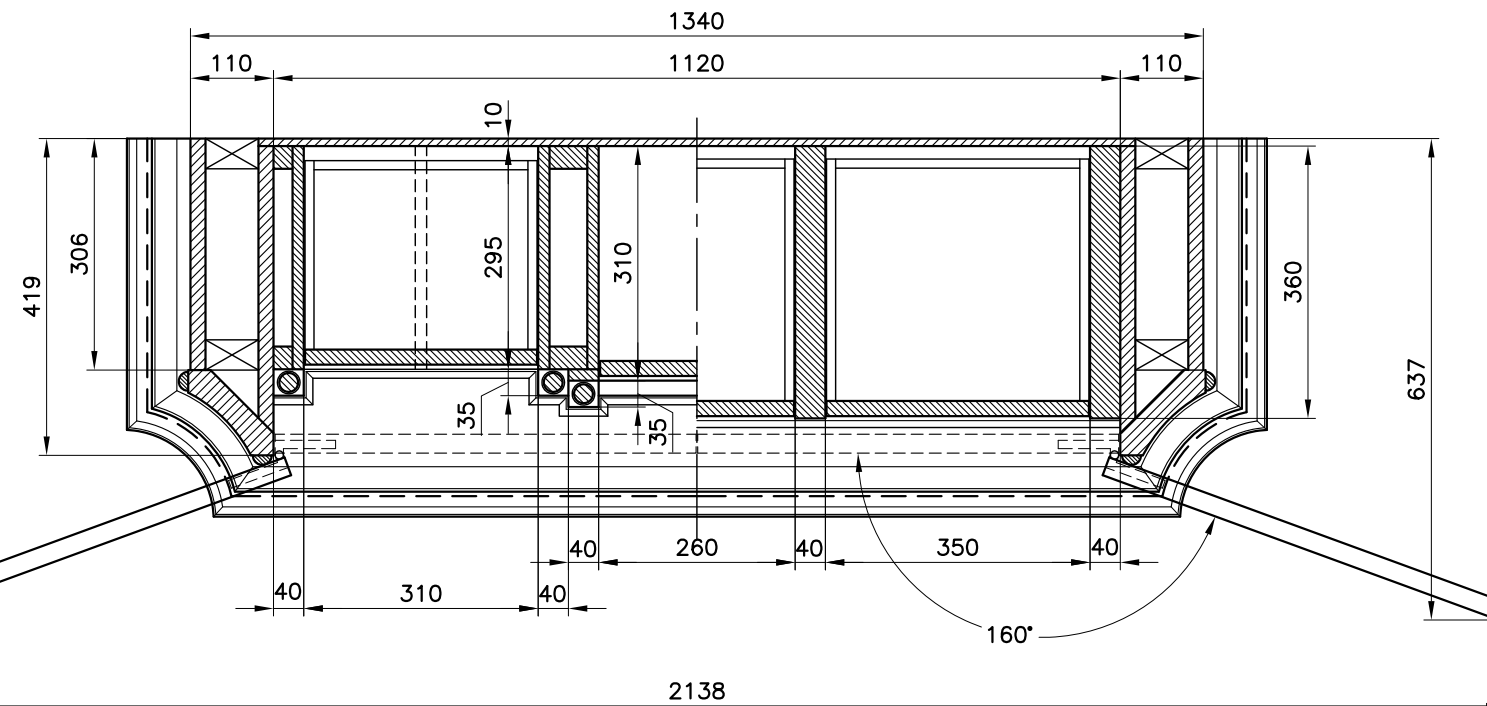
SEZIONE E-E
