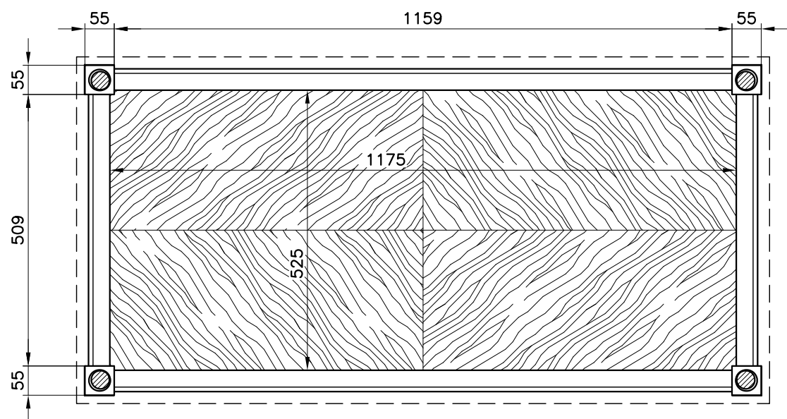
SEZIONE ORIZZ.
