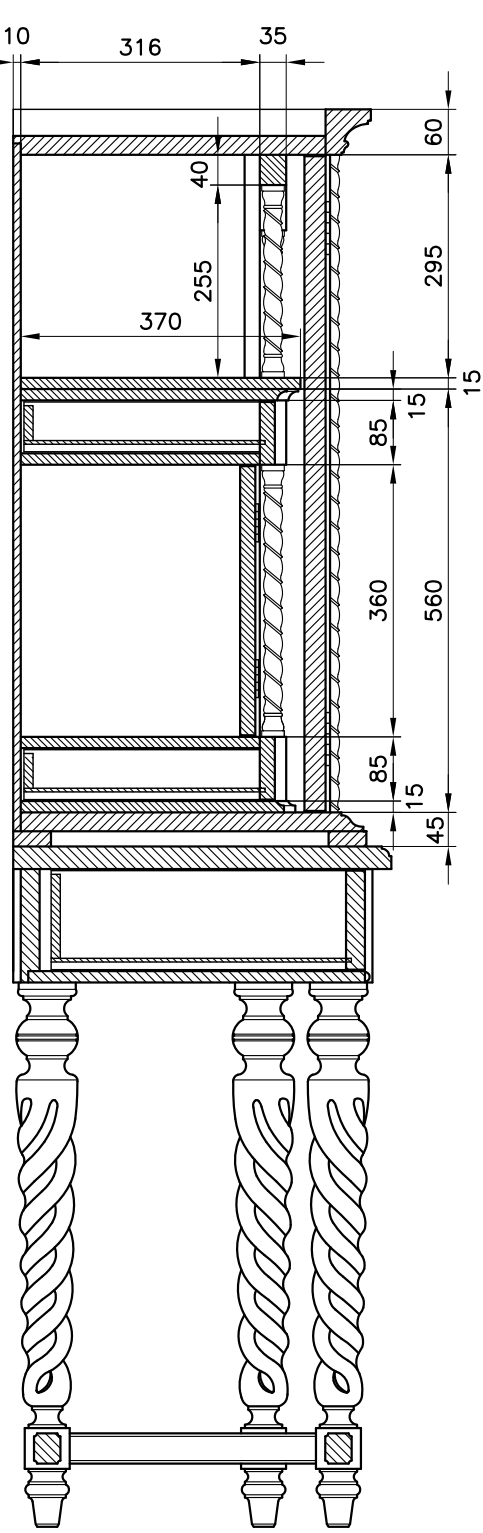
SEZIONE B-B
