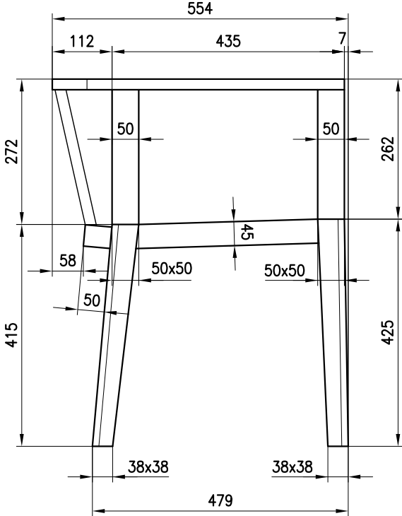
FIANCO
