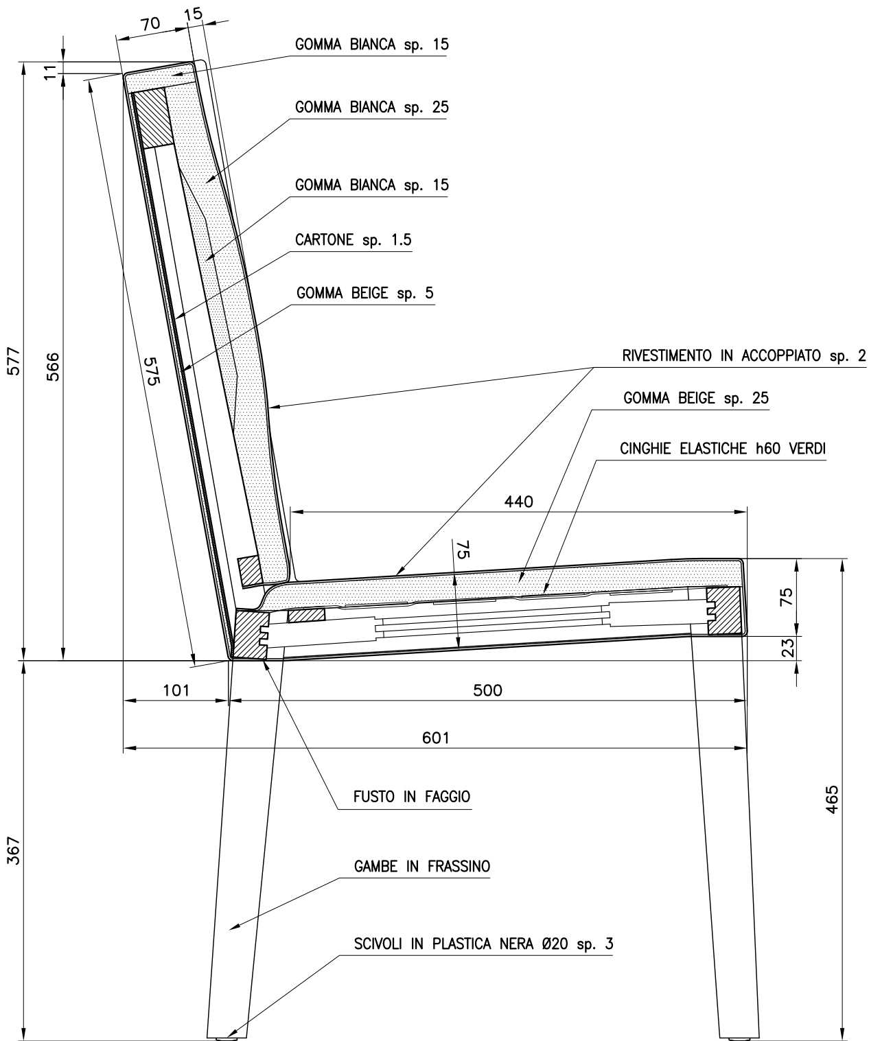
SEZIONE VERTICALE
