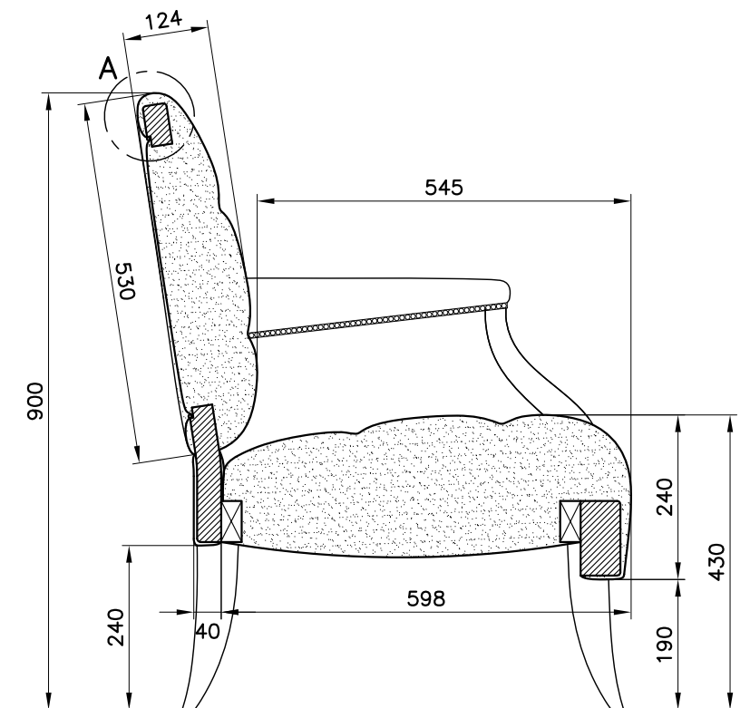
SEZIONE VERTICALE
