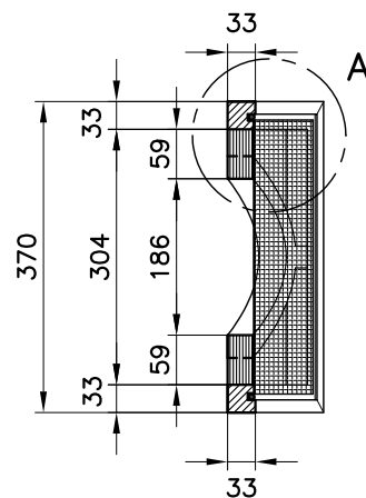
PART. A scala 1:2
