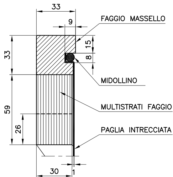
PART. A scala 1:2
