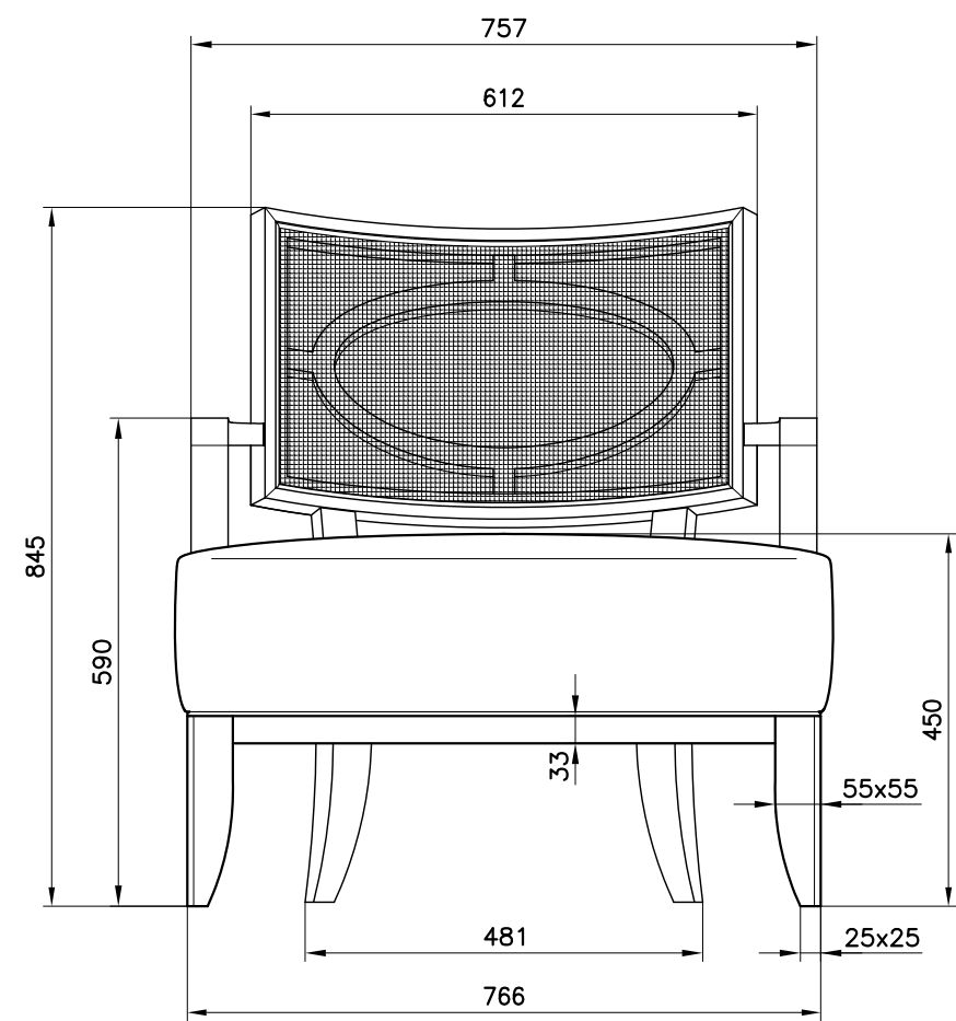
PROSPETTO
