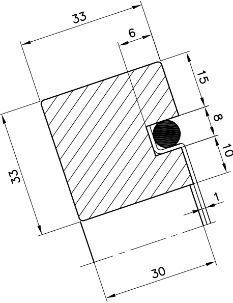
PART. A scala 1:1
