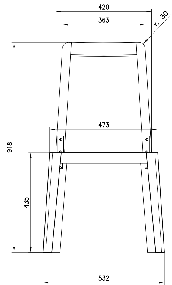
PROSPETTO
