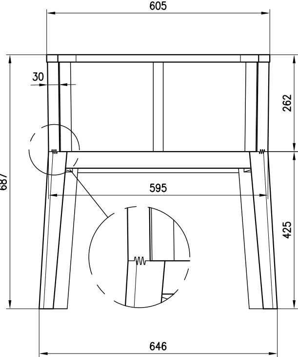
PROSPETTO
