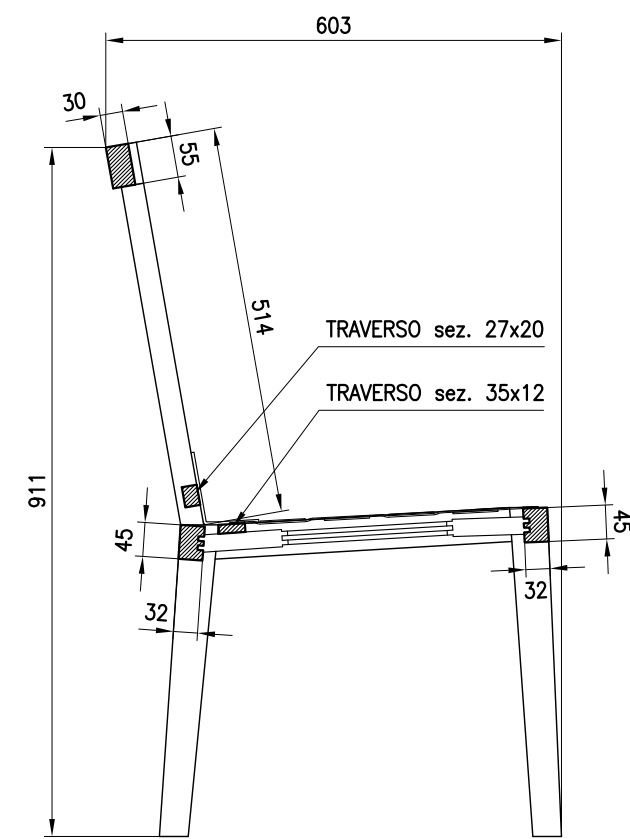
SEZIONE VERTICALE
