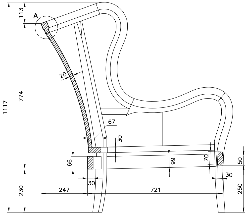
SEZIONE VERTICALE
