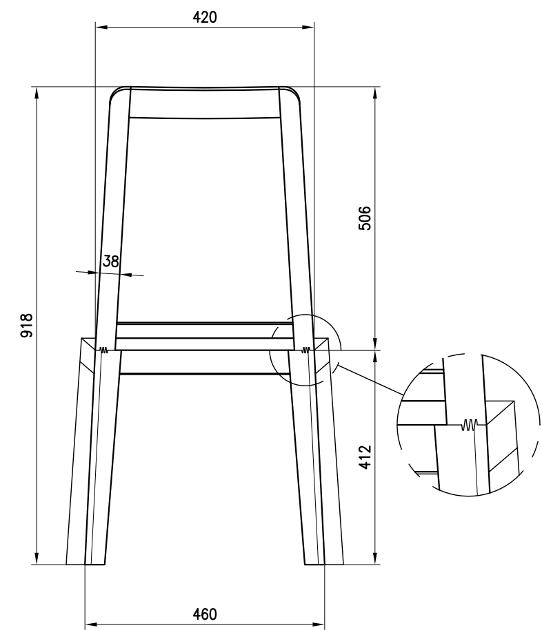
VISTA POSTERIORE
