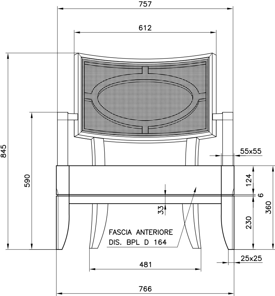
PROSPETTO
