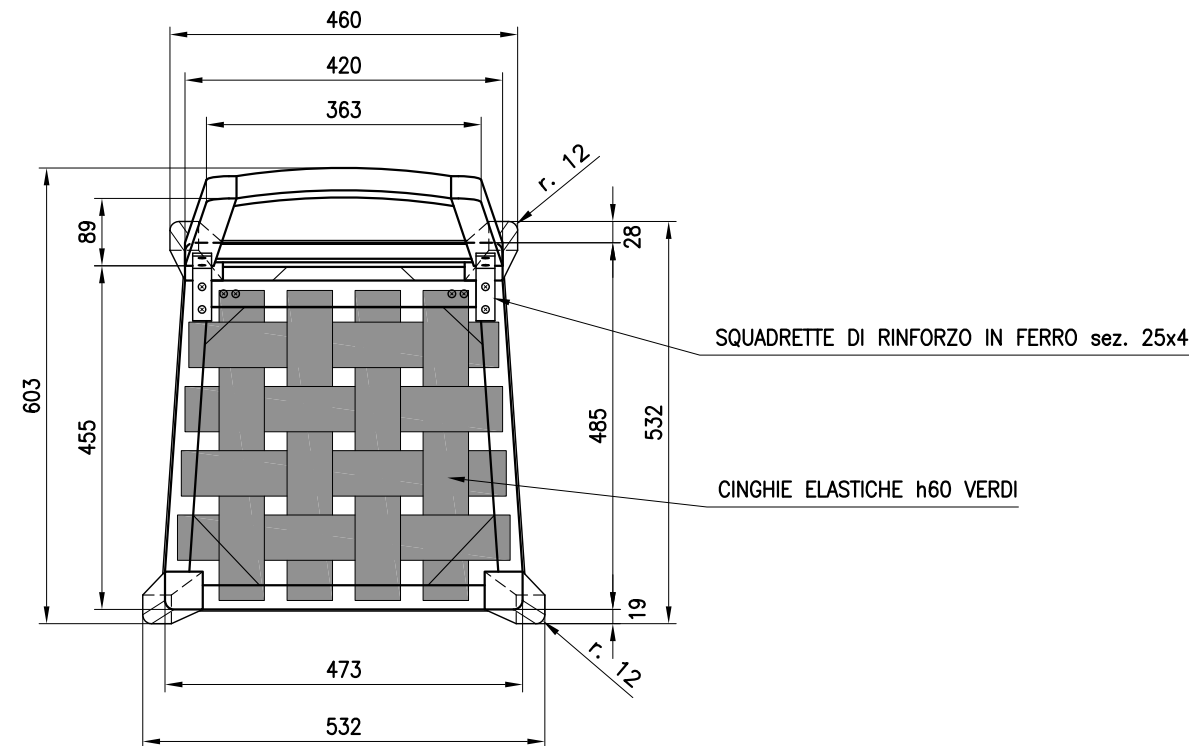
PIANTA
