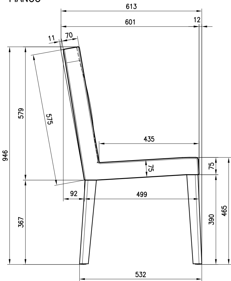
FIANCO
