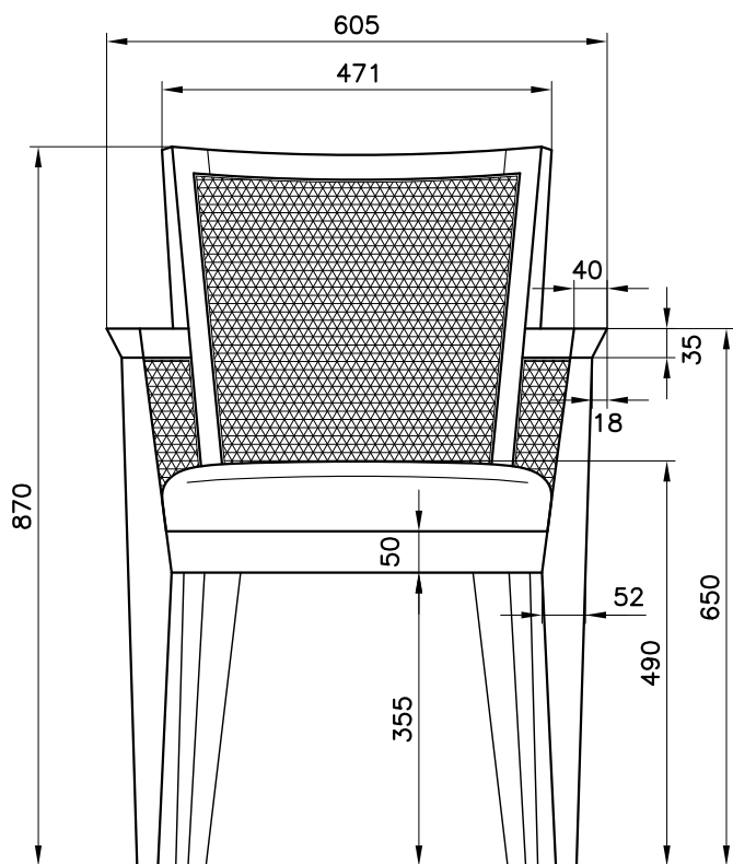
FRONTE
