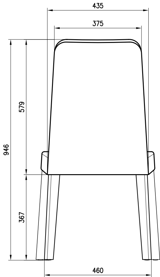
VISTA POSTERIORE
