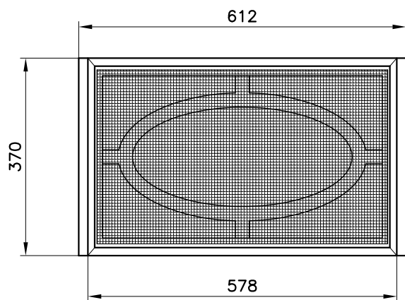
FRONTE
