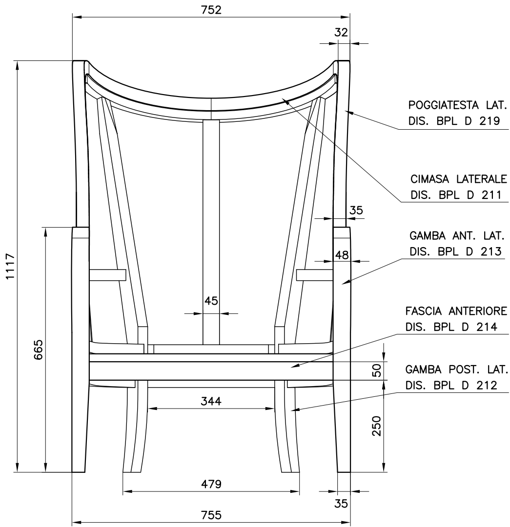
PROSPETTO
