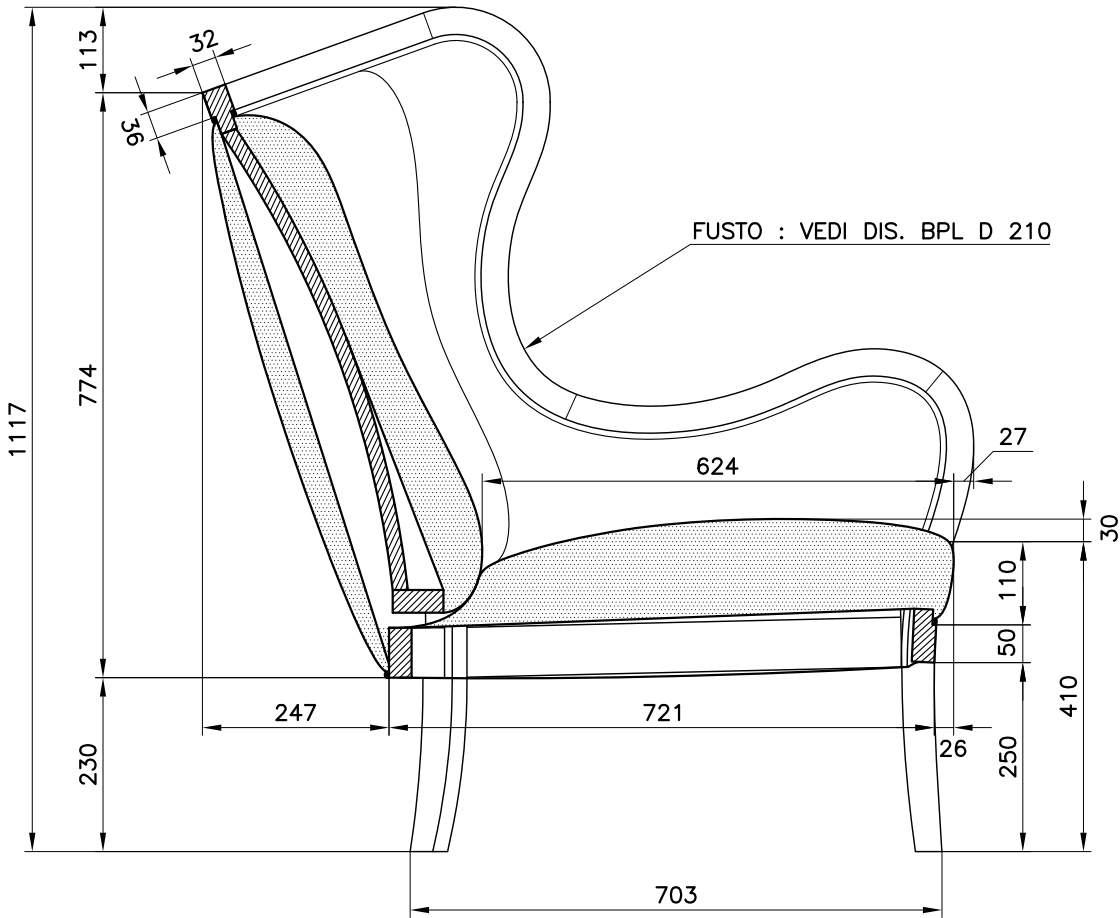
SEZIONE VERTICALE
