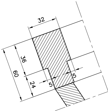
PART. A scala 1:2
