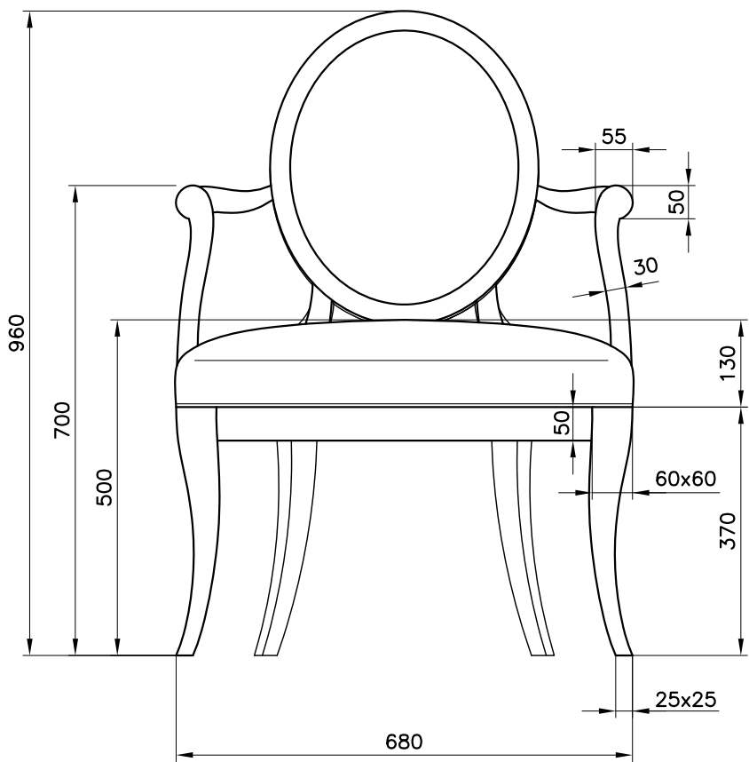
FRONTE
