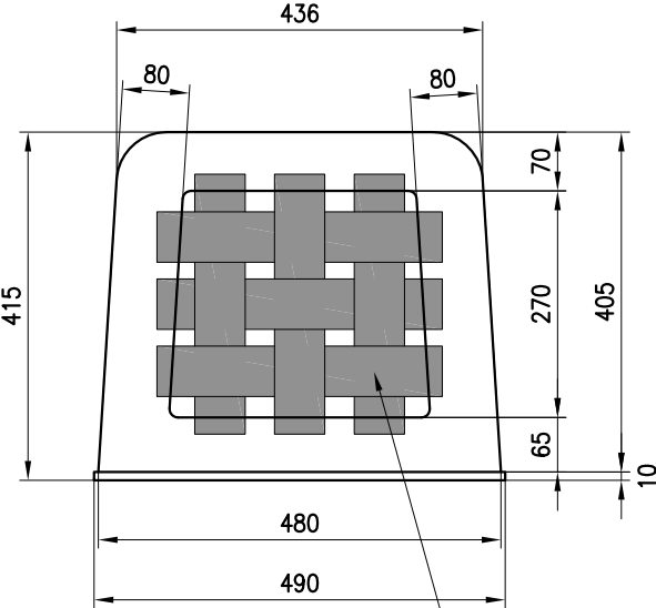
PIANTA SEDILE
