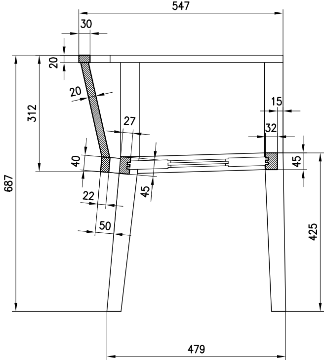
SEZIONE VERTICALE
