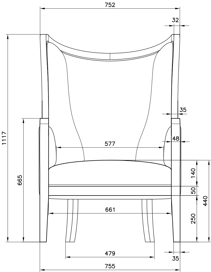
PROSPETTO
