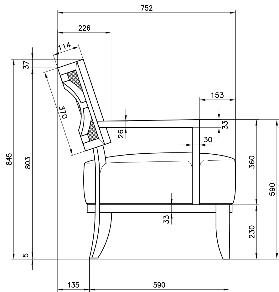
FIANCO
