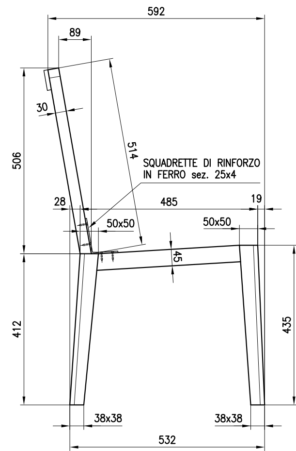
FIANCO
