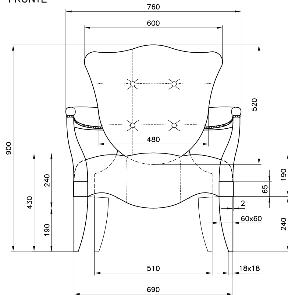
FRONTE
