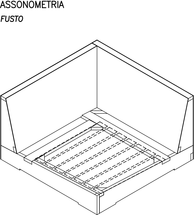
FUSTO SENZA UN COMPENSATO SU SCHIENALE
