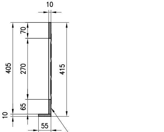
SEZIONE SEDILE
