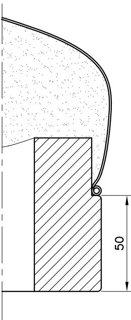
PART. B scala 1:2
