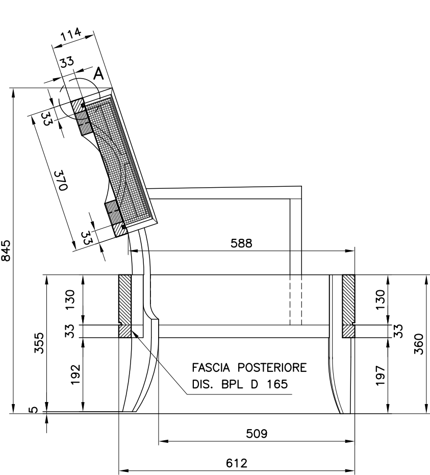
SEZIONE VERTICALE
