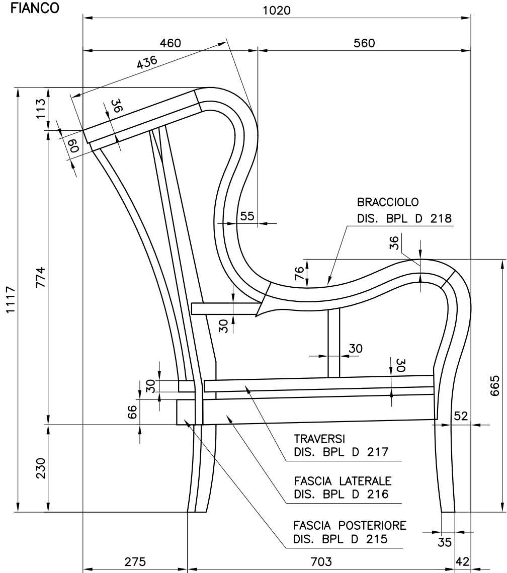
FIANCO
