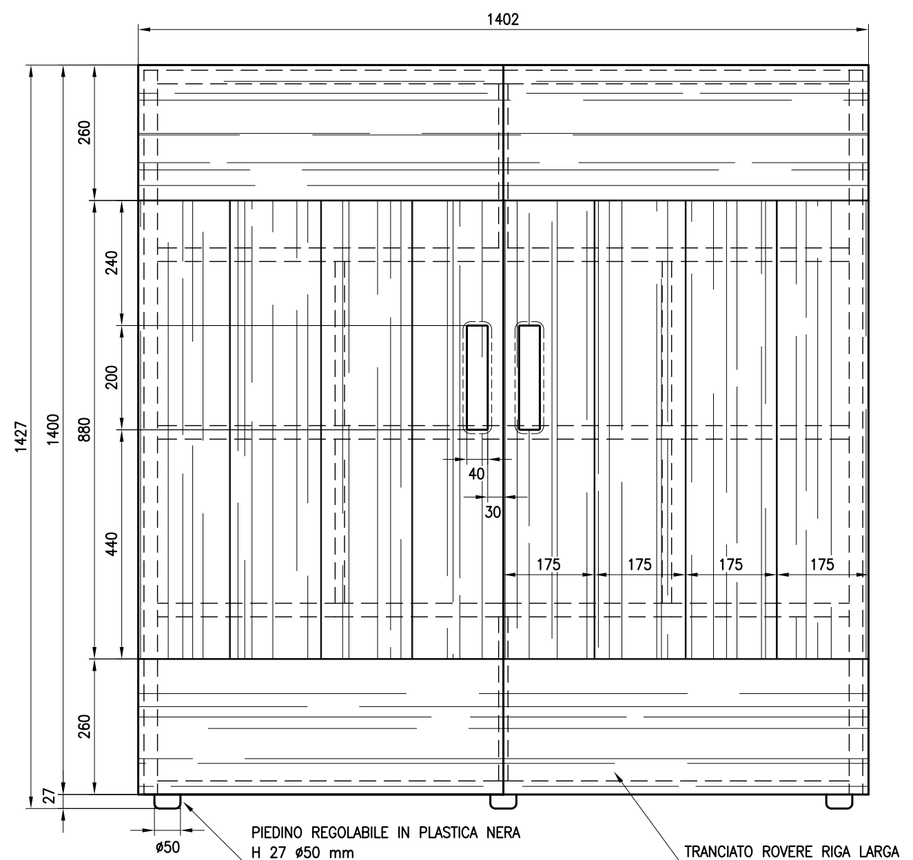
FRONTE
