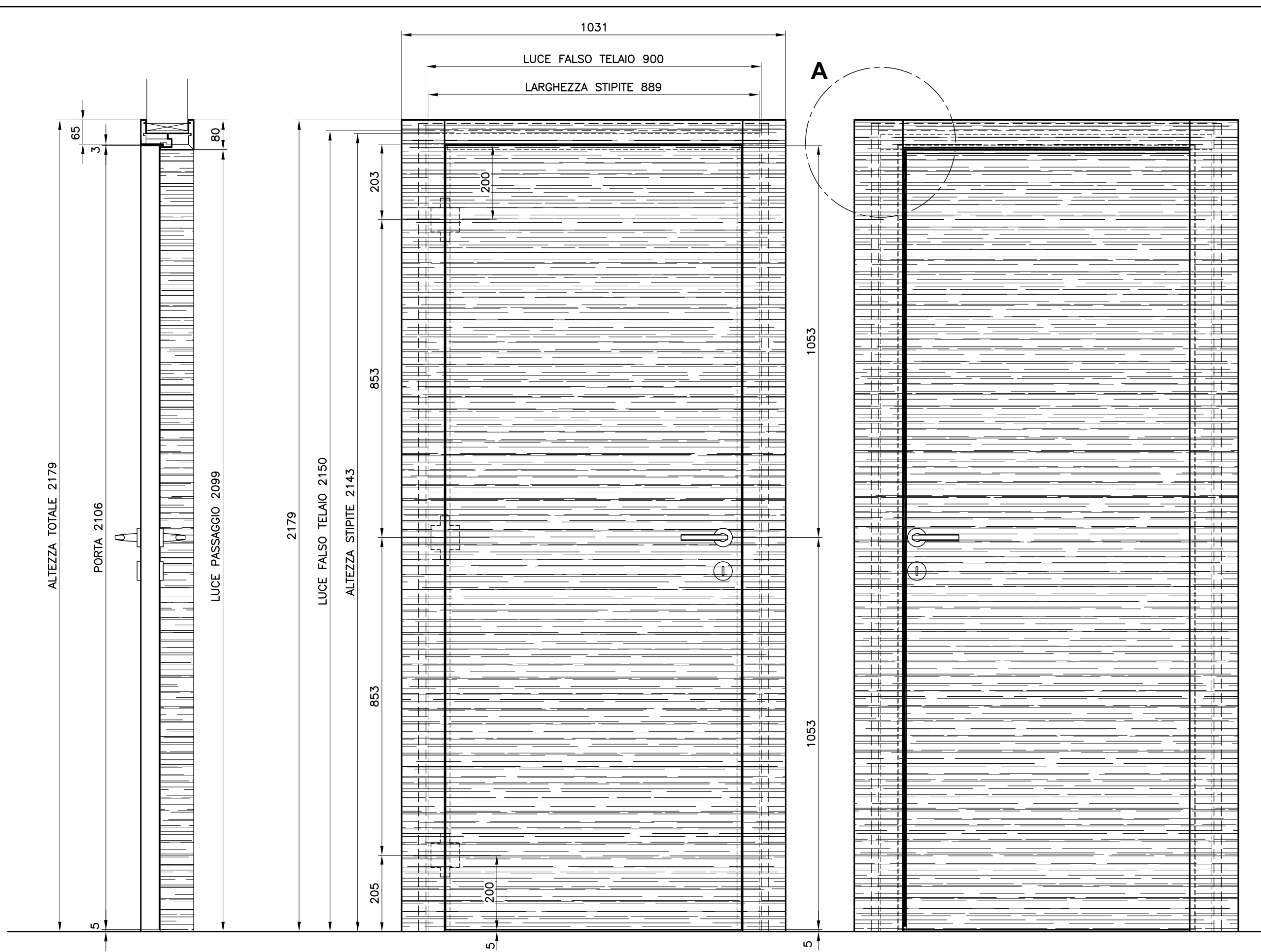
SEZIONE VERTICALE
