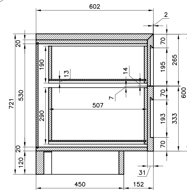
SEZIONE B-B scala 1:10
