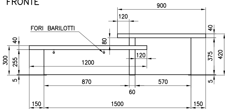
FRONTE
