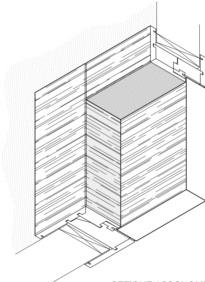
SEZIONE ASSONOMETRICA PARTICOLARE A
