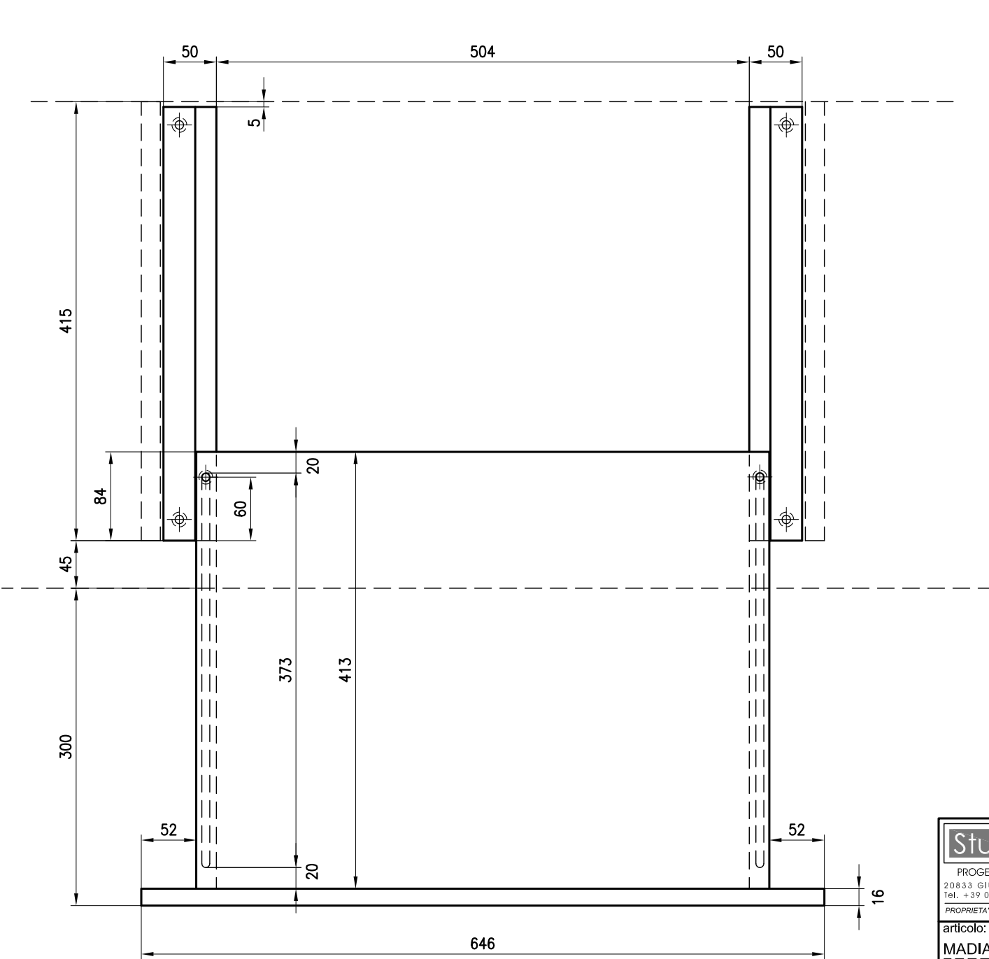
PIANTA (APERTO)
