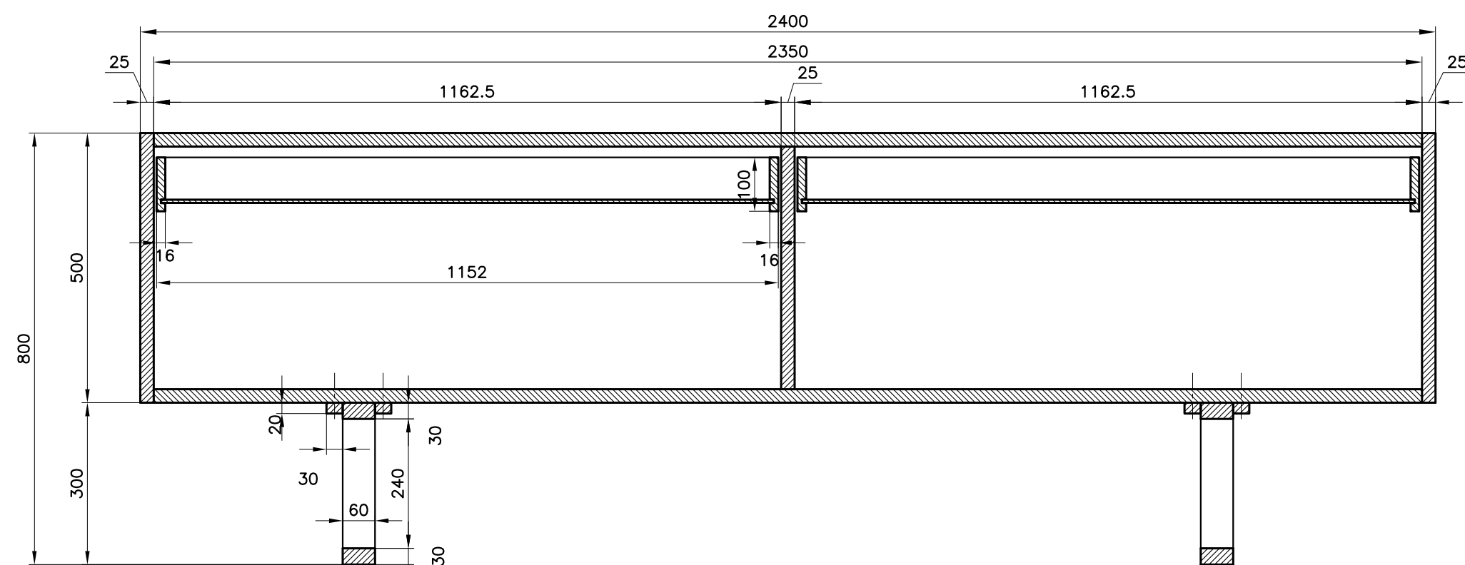
SEZIONE A-A scala 1:10
