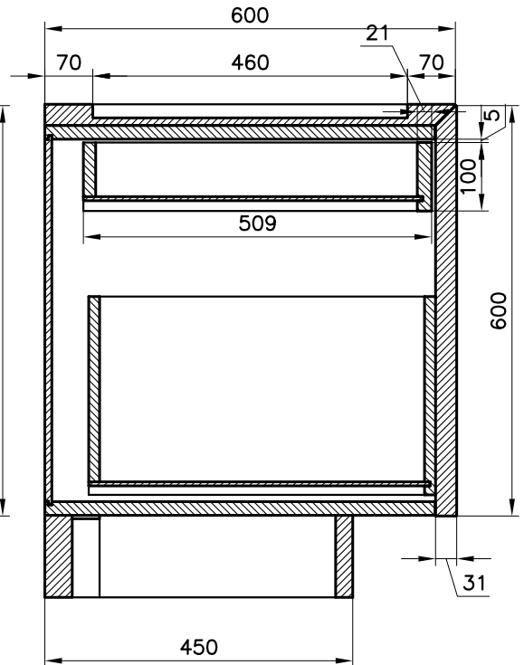
SEZIONE C-C scala 1:10
