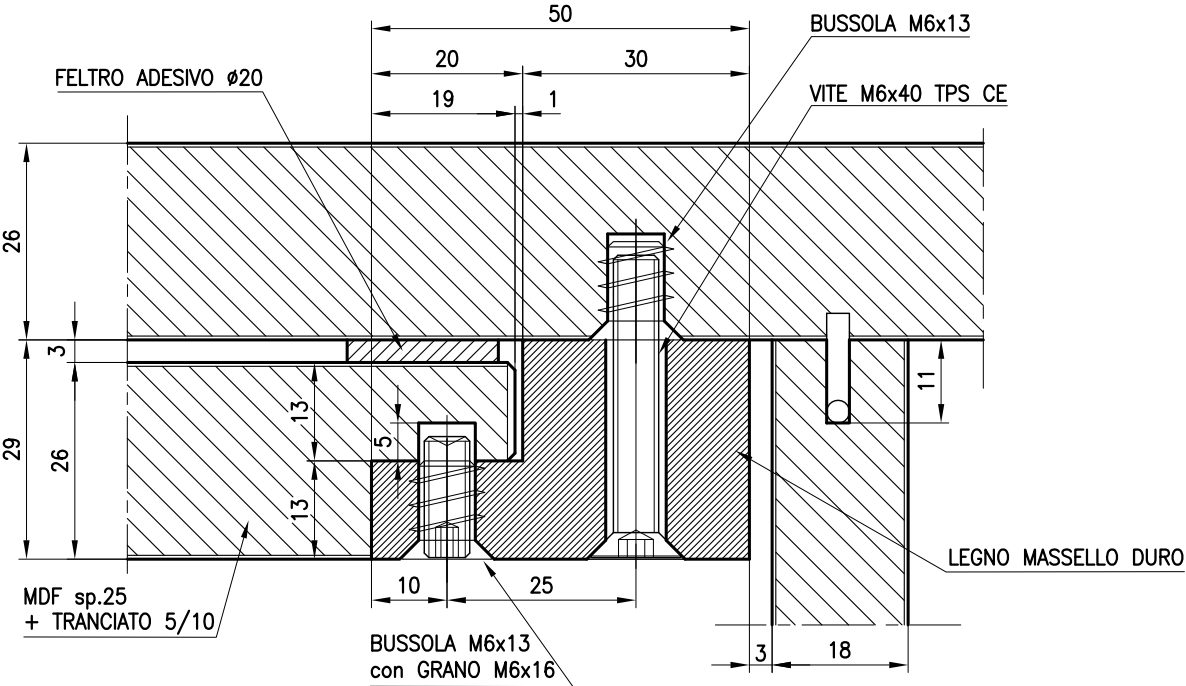
SEZIONE FRONTALE scala 1:1
