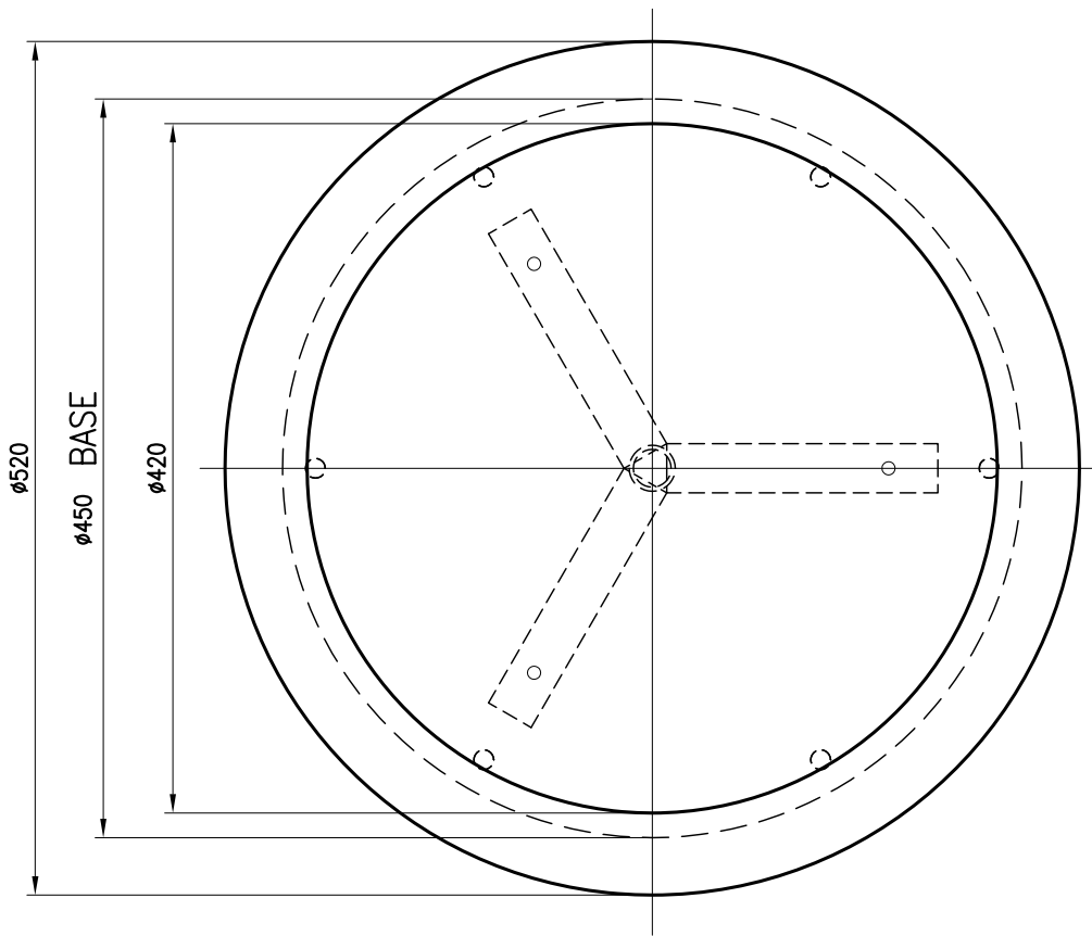
PART. A scala 1:1
