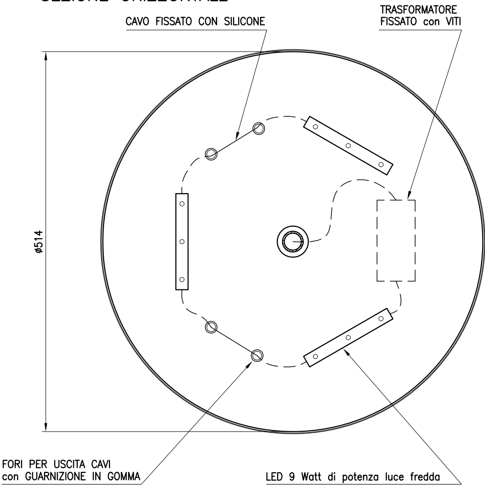
SEZIONE ORIZZONTALE
