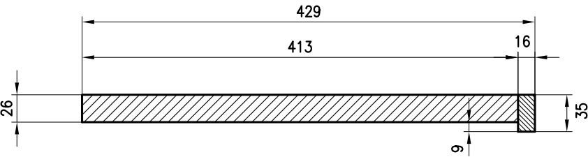
SEZIONE TIRETTO
