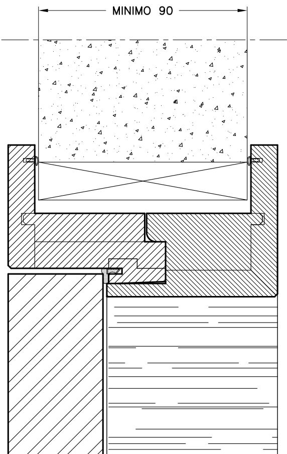
SEZIONE VERTICALE scala 1:2
