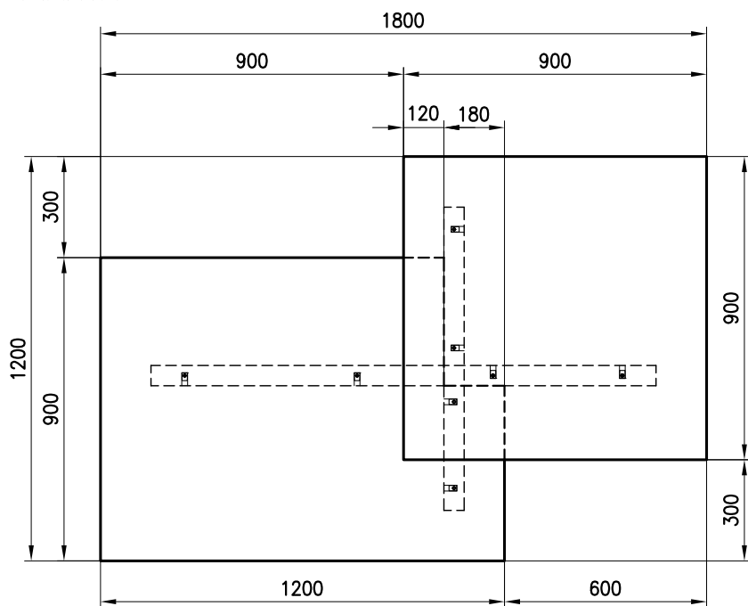
PIANTA
