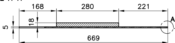
SEZIONE A-A
