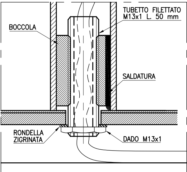
PART. A scala 1:1
