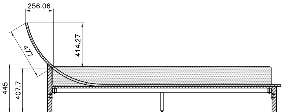
SEZIONE VERTICALE
