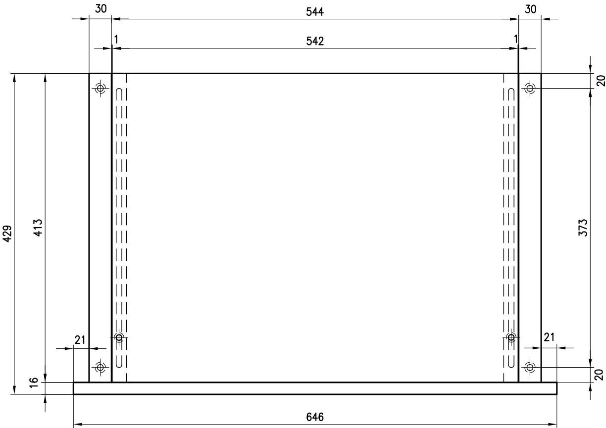
PIANTA (CHIUSO)
