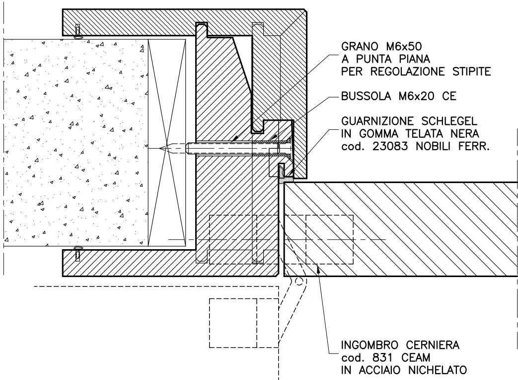
SEZIONE ORIZZONTALE scala 1:2
