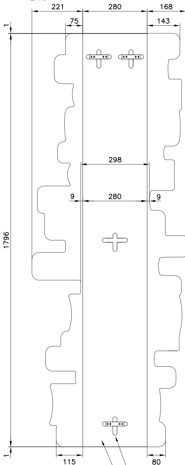
PART. A scala 1:1
