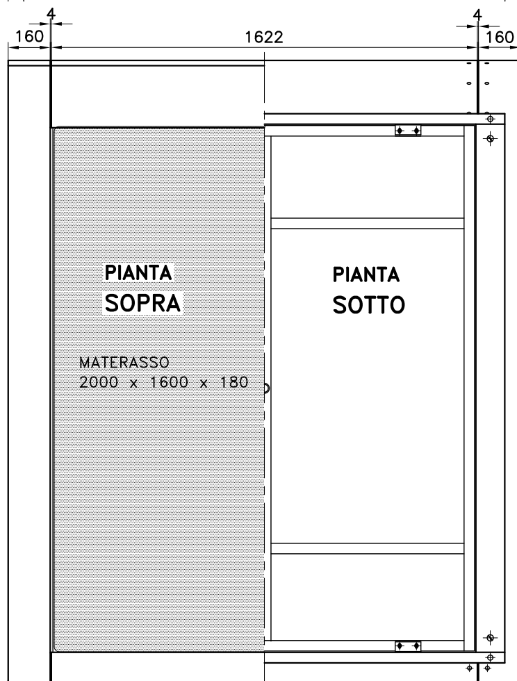
PARTICOLARE scala 1:2
