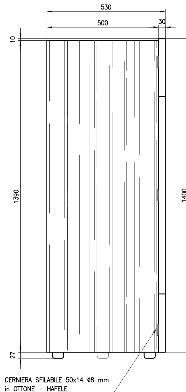
FIANCO
