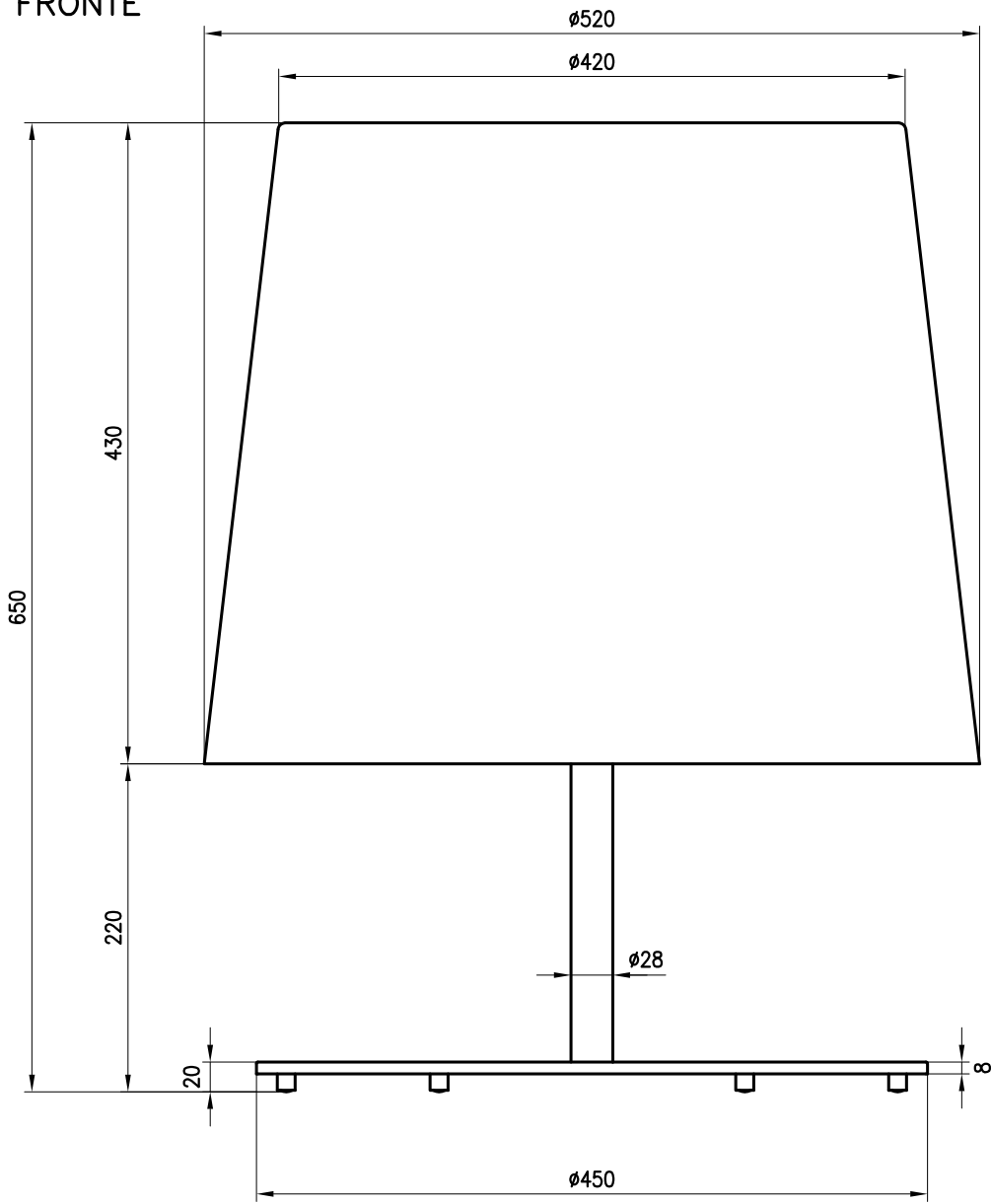
FRONTE
