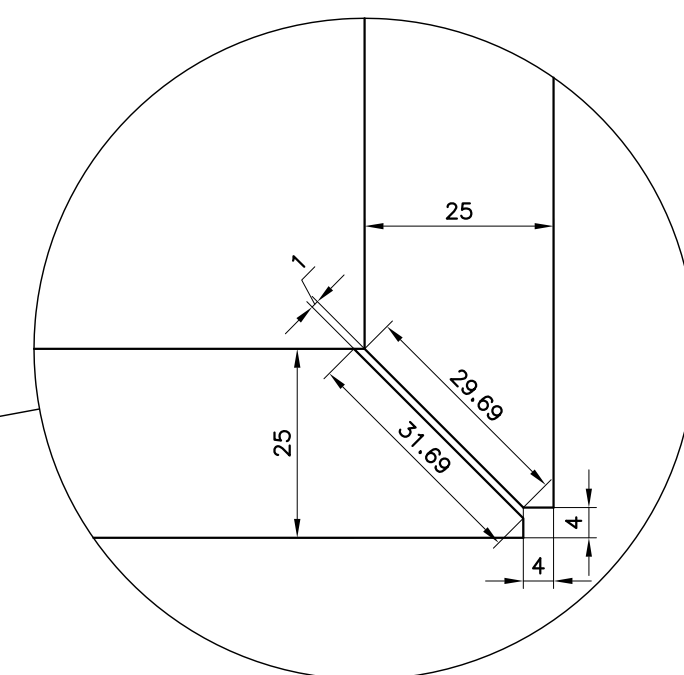
PARTICOLARE scala 1:2
