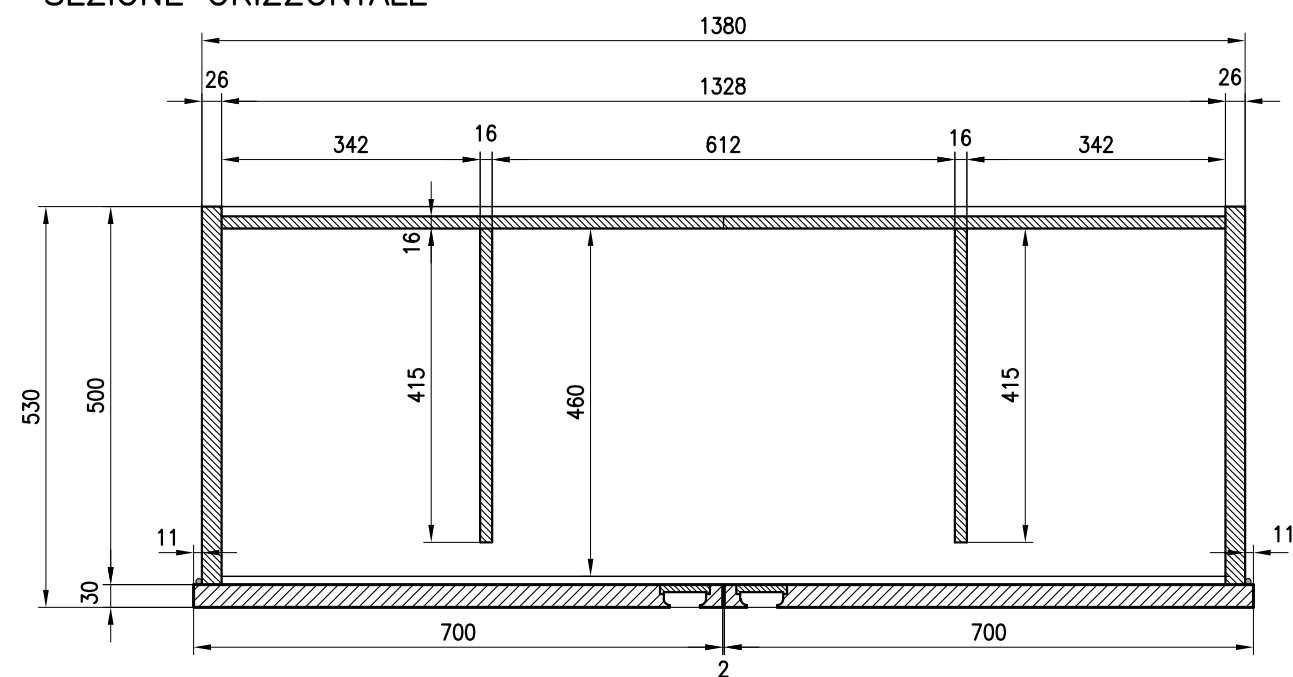
SEZIONE ORIZZONTALE
