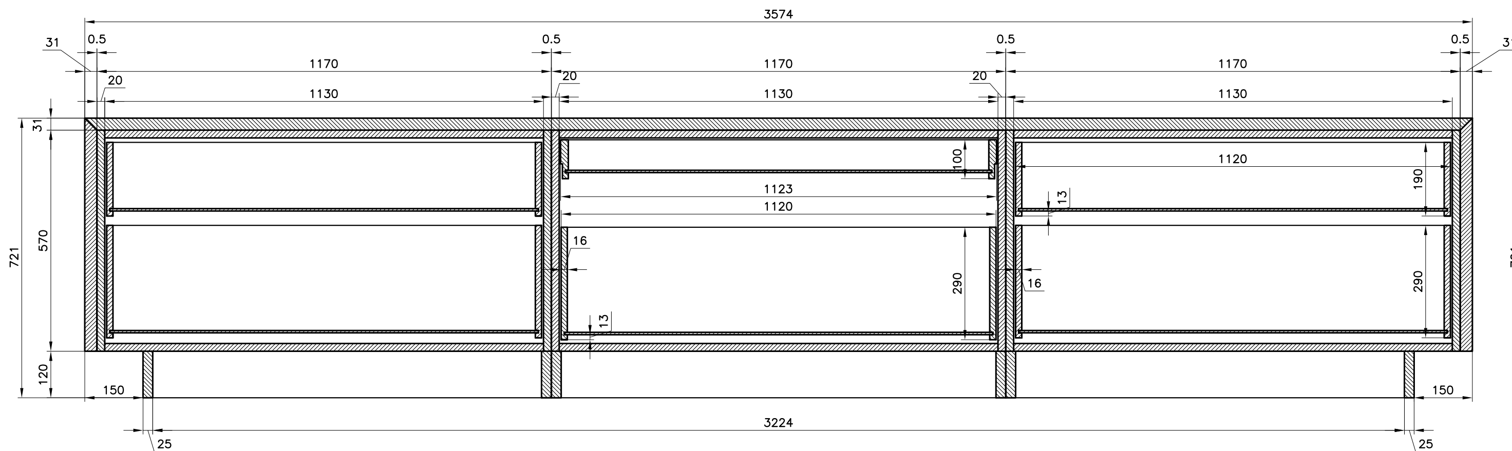
SEZIONE A-A scala 1:10
