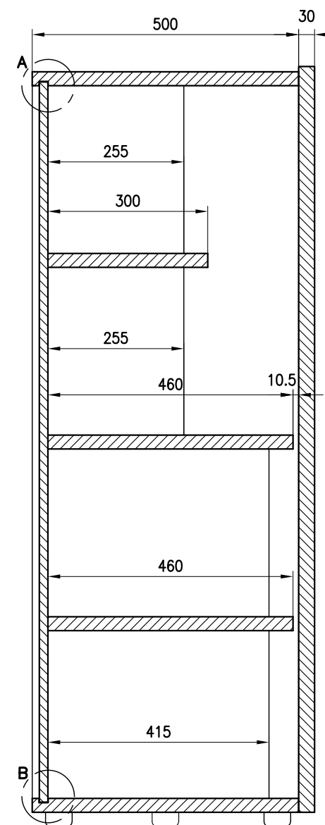
SEZIONE VERTICALE
