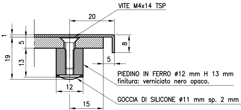
PART. B scala 1:1
