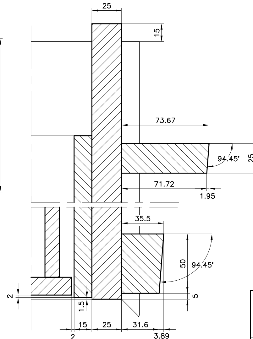
PART. C – D scala 1:2
