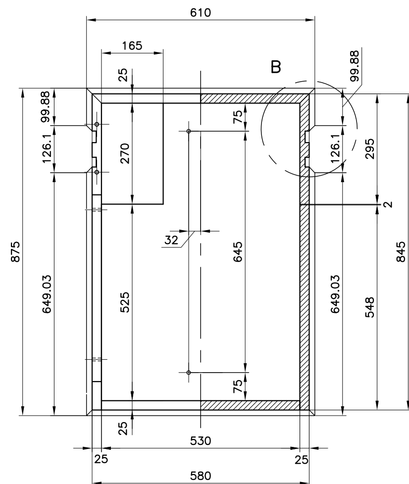
SEZIONE A-A
