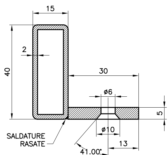
SEZ. A-A scala 1:1
