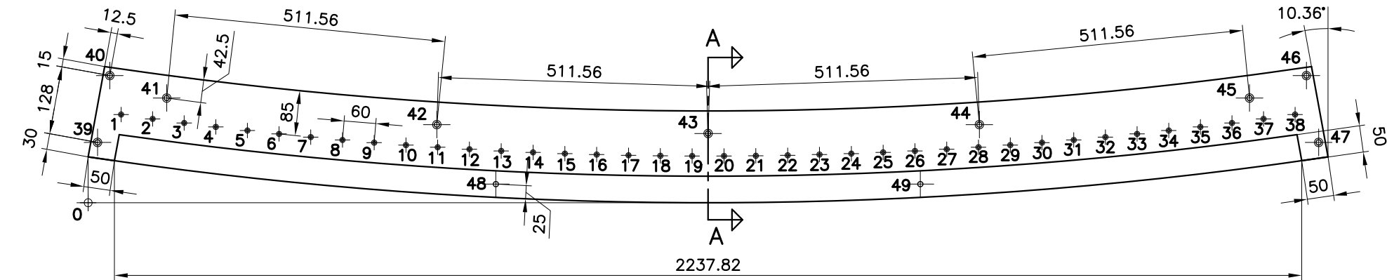
PIANTA
