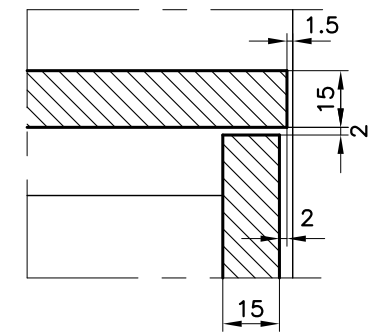
PART. B scala 1:2
