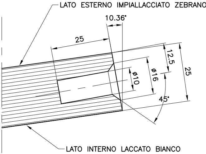
SEZ. A-A scala 1:1
