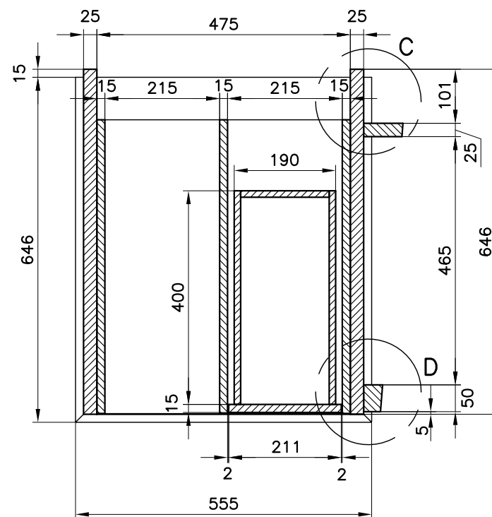
SEZIONE A-A
