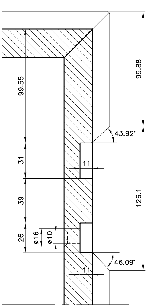
PART. C scala 1:2
