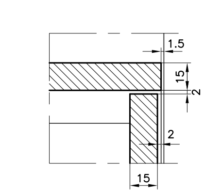
PART. B scala 1:2
