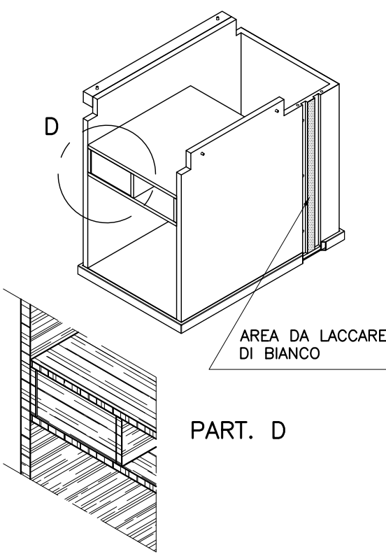
VISTA ASSONOMETRICA
