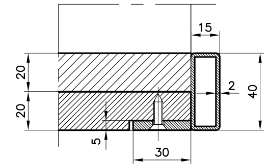
PART. B scala 1:2
