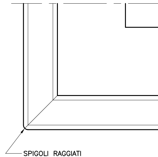
SEZ. A-A scala 1:1
