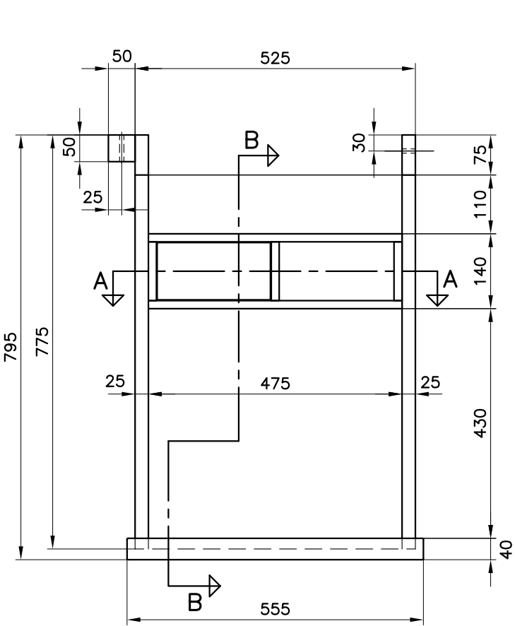
FRONTE INT.
