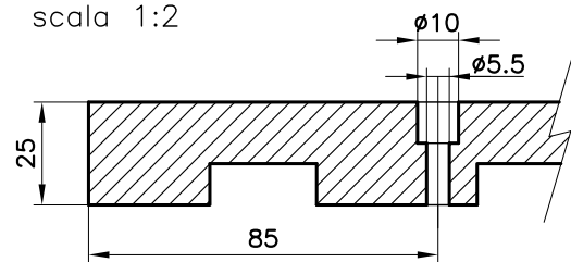
SEZIONE FORI DAL n°1 AL n°38 PER FIBRE OTTICHE scala 1:2
