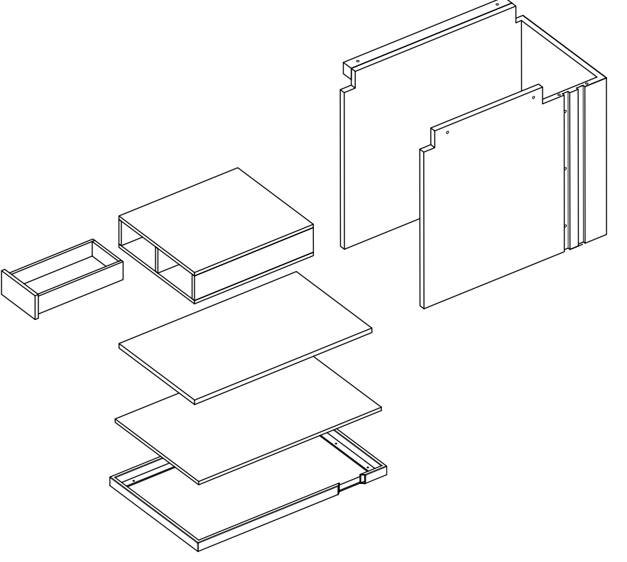
ESPLOSO COMPONENTI
