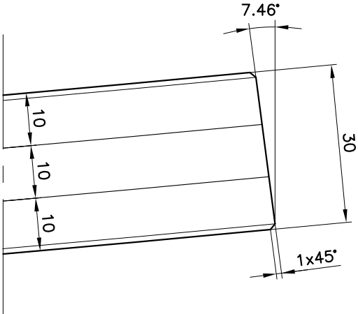
PART. B scala 1:1
