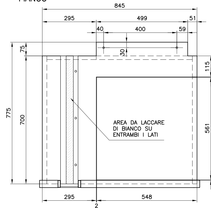
FIANCO
