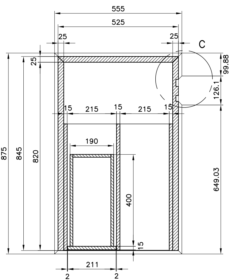
SEZIONE A-A
