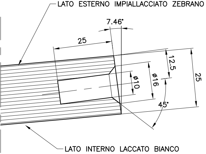
SEZ. B-B scala 1:1
