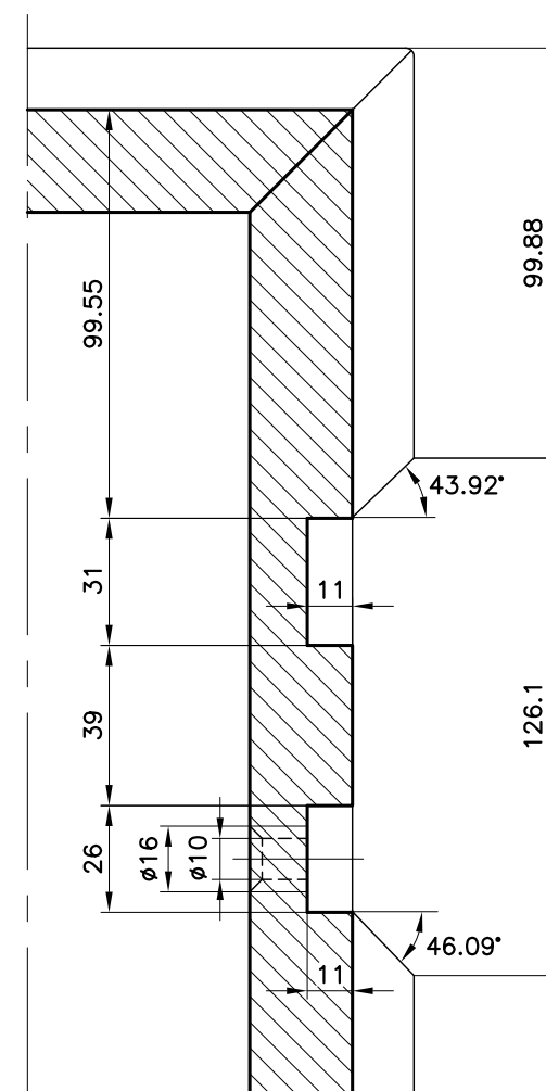
PART. B scala 1:2
