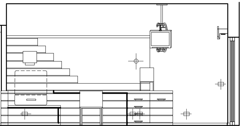
ALZATO B
